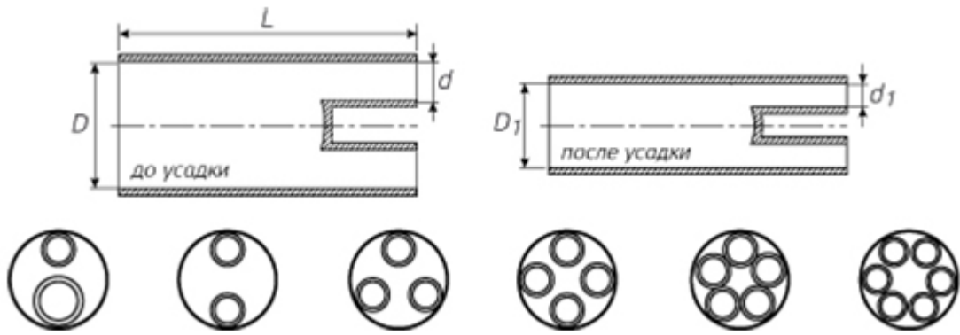
Размеры (мм)
