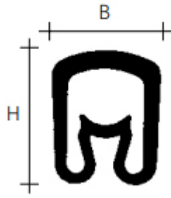
Размеры (мм)
