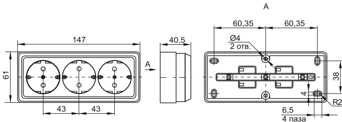
Рисунок 7. Розетки РС23-3-ОБ; РС23-3-ОК; РС23-3-ОС; РС23-3-ОД.
