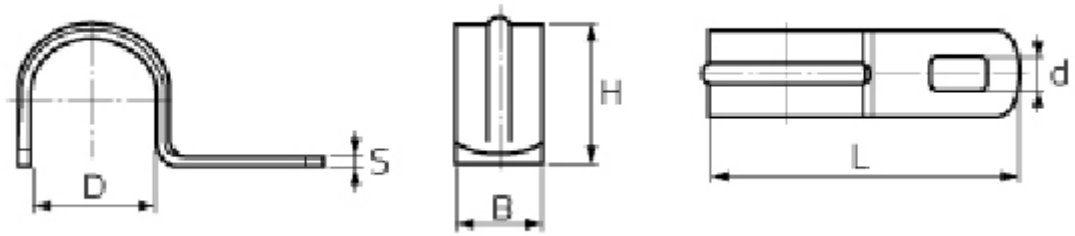
Размеры (мм)
