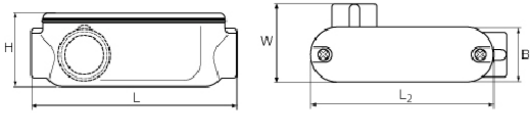
Размеры (мм)
