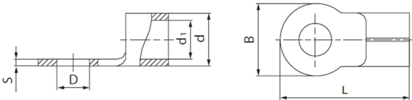
Размеры (мм)
