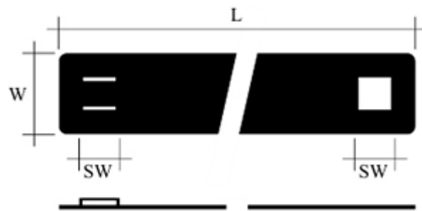
Размеры (мм)
