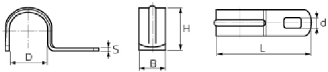
Размеры (мм)
