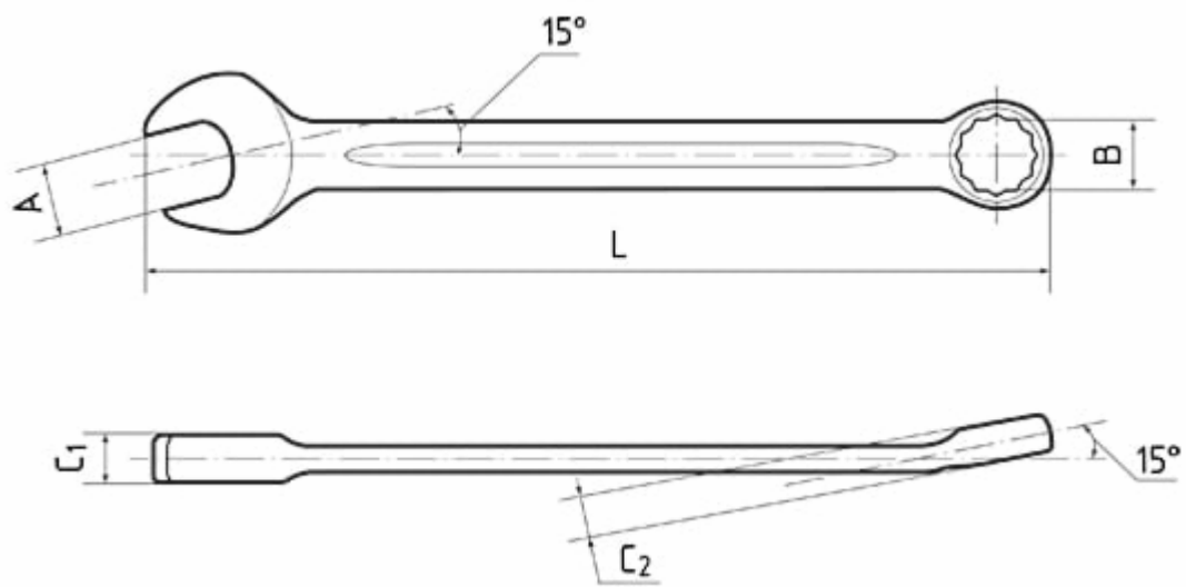
Размеры (мм)
