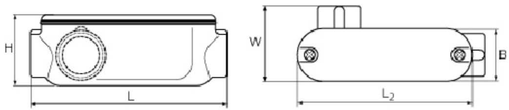
Размеры (мм)
