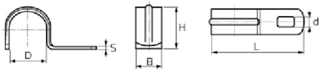
Размеры (мм)
