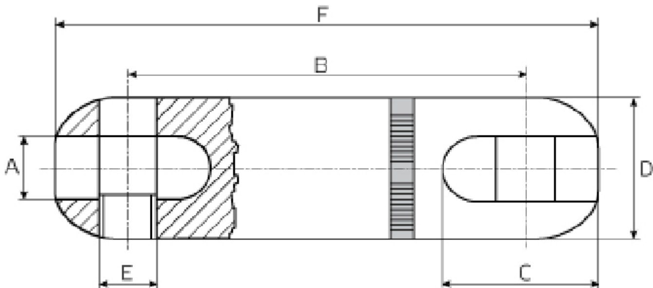
Размеры (мм)
