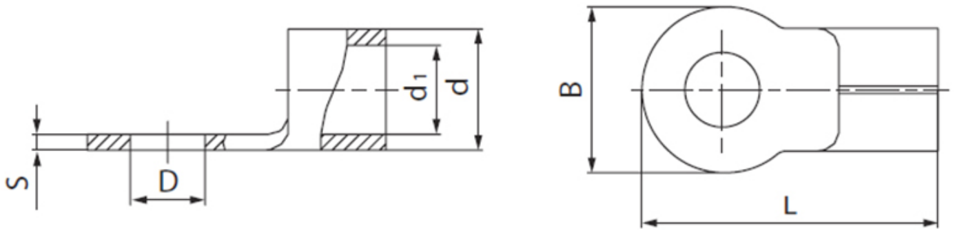
Размеры (мм)
