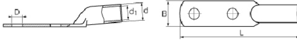
Размеры (мм)
