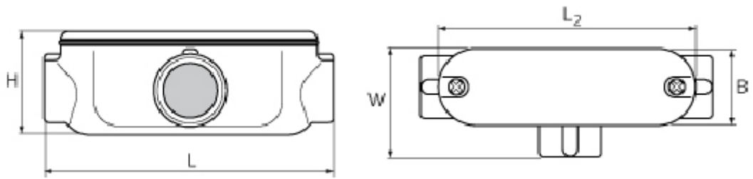
Размеры (мм)
