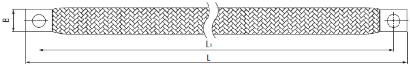
Размеры (мм)
