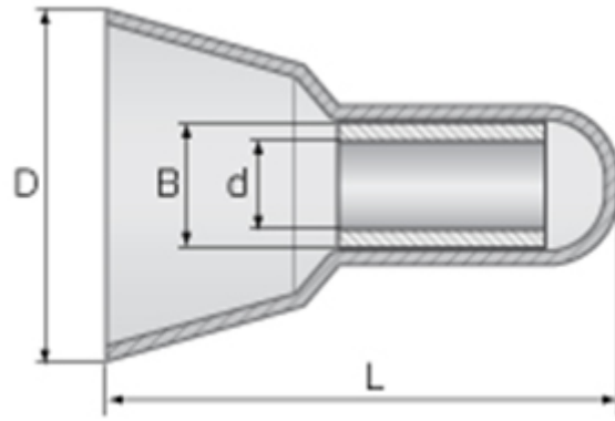
Размеры (мм)
