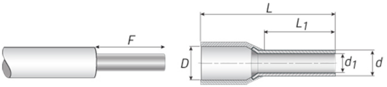
Размеры (мм)
