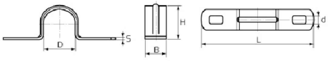
Размеры (мм)
