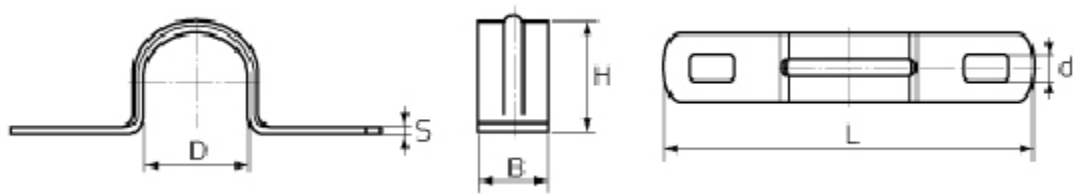
Размеры (мм)
